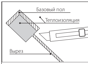
Рисунок 17. Подготовка теплоизоляции в месте размещения датчика температуры.
