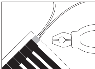
Рисунок 19. Подключение к нагревательной пленке установочных проводов.
