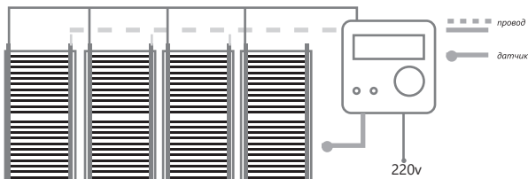
рис.4 (схема подключения)
