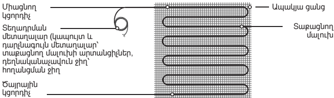
Նկ 1. Ներքևակի կառուցվածքը
