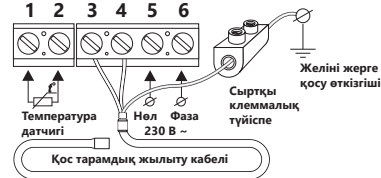
2-сур. Төсенішті электр желісіне қосу схемасы
