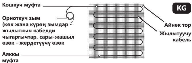
1-сүр. Маттын конструкциясы
