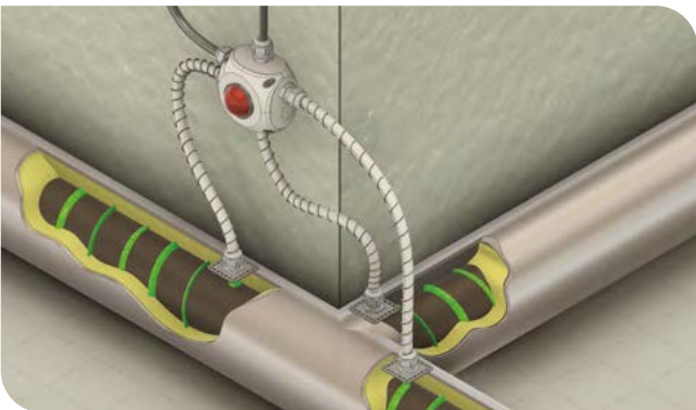
Индикаторный элемент
