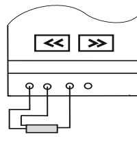
Подключение тсм Pt100 и 50M
